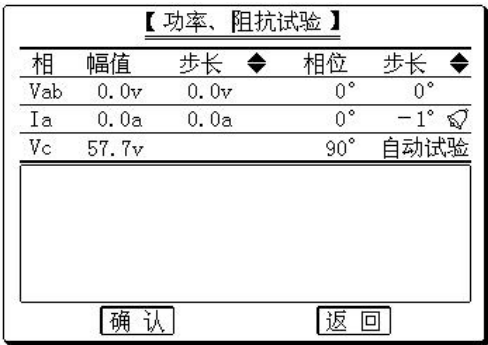
功率阻抗
